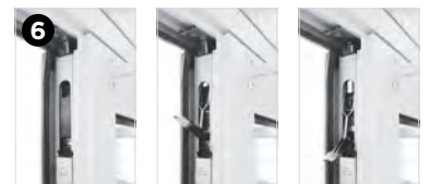
Verrous haut et bas intégrés dans les profils (hors vantaill principal pourvu d'une serrure)
